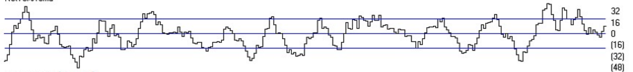
UKA %NNH25 (+ 5ma)
