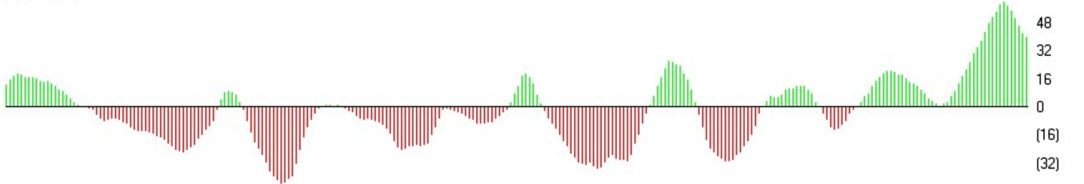
CP PriceOsc
